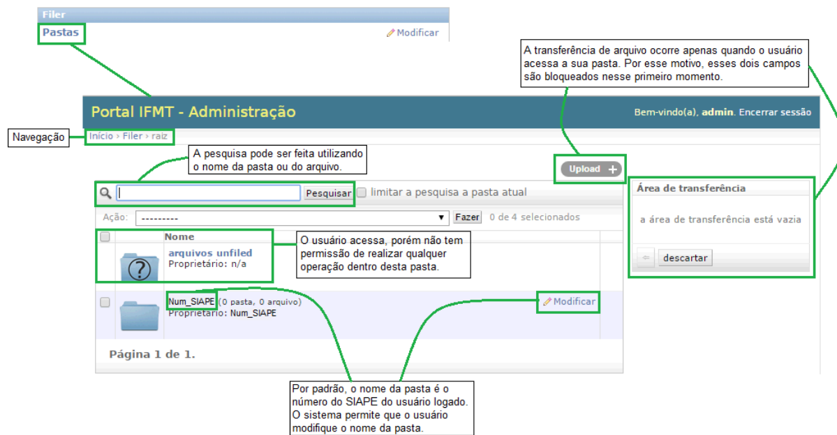
Figura 8 - Tela inicial do gerenciador de arquivos
