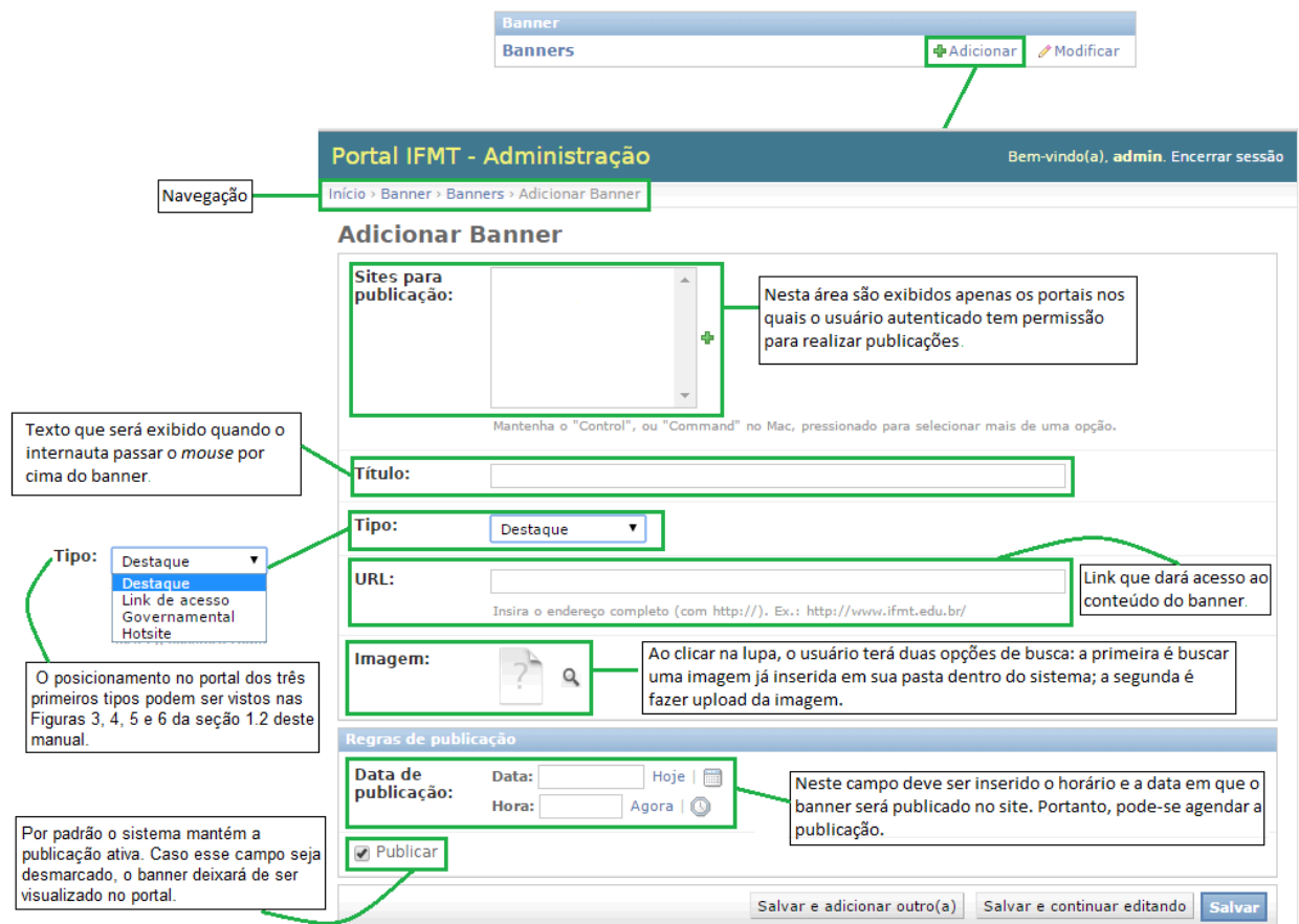
Figura 40 - Tela de cadastro dos banners
